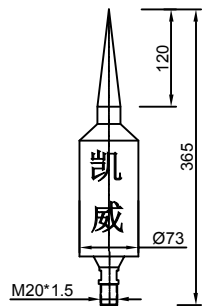
艾力高提前放电避雷针 SI25
